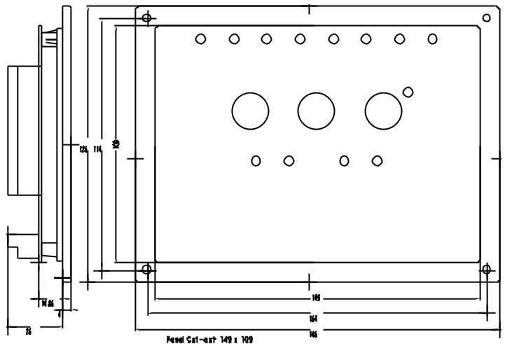
Fig. 3 Dimensions (mm)
