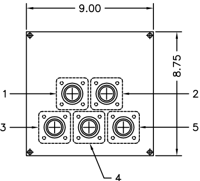
PANEL (SCALE: 3=1)
