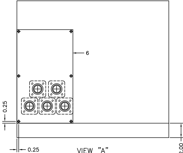
VIEW "A" (SCALE: 3=1)
