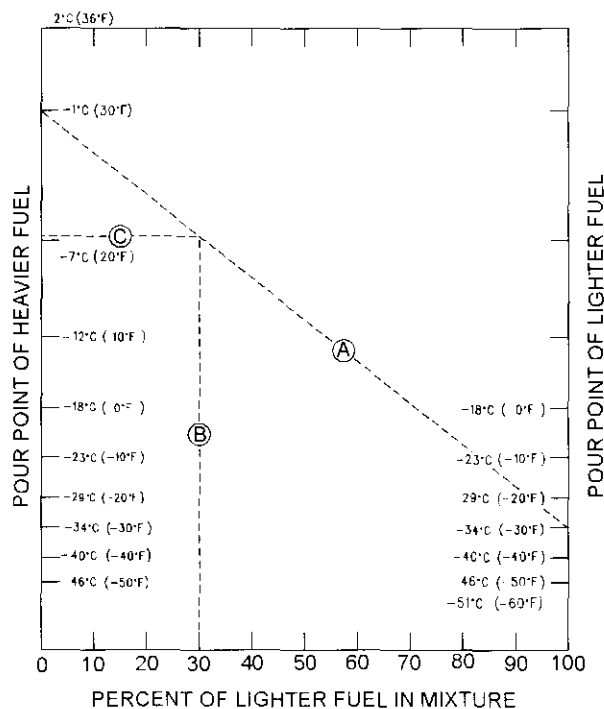
Illustration 6 g01180699 Pour point of fuel mixtures
